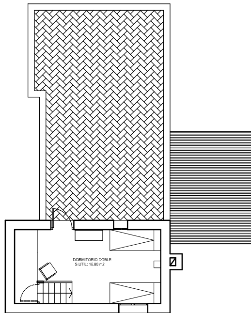
DISTRIBUCION PLANTA ALTA
